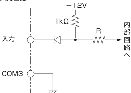
入力回路
