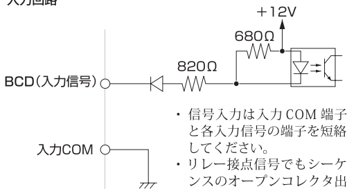
入力回路
