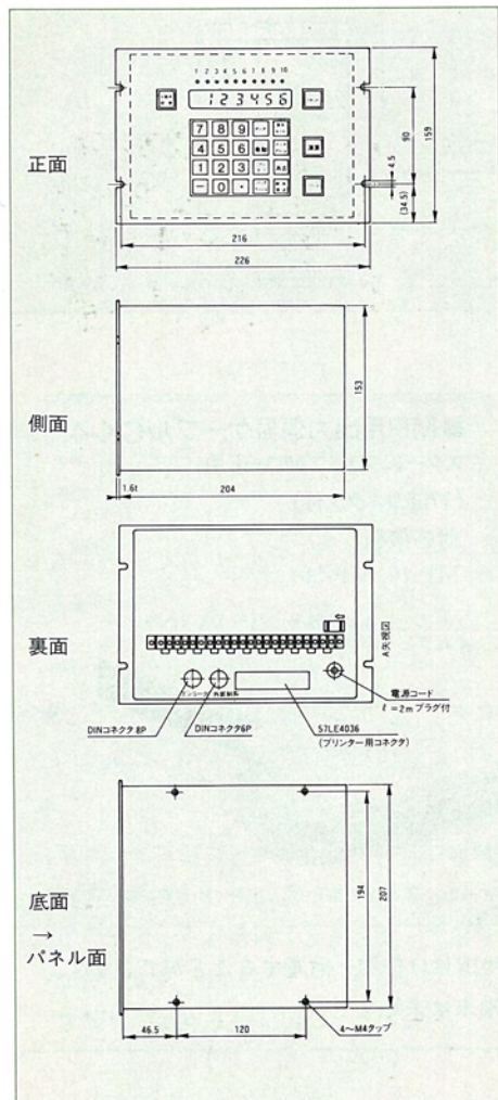
■10ポイント出力カウンタ<Tシリーズ>外形図
