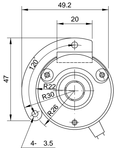
スプリングフランジ取付図
