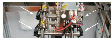
ヘッド前後に2個ずつ搭載された冷却ファン(白矢印)
